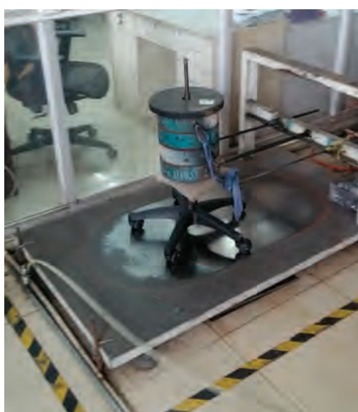
의자오발 하중실험
